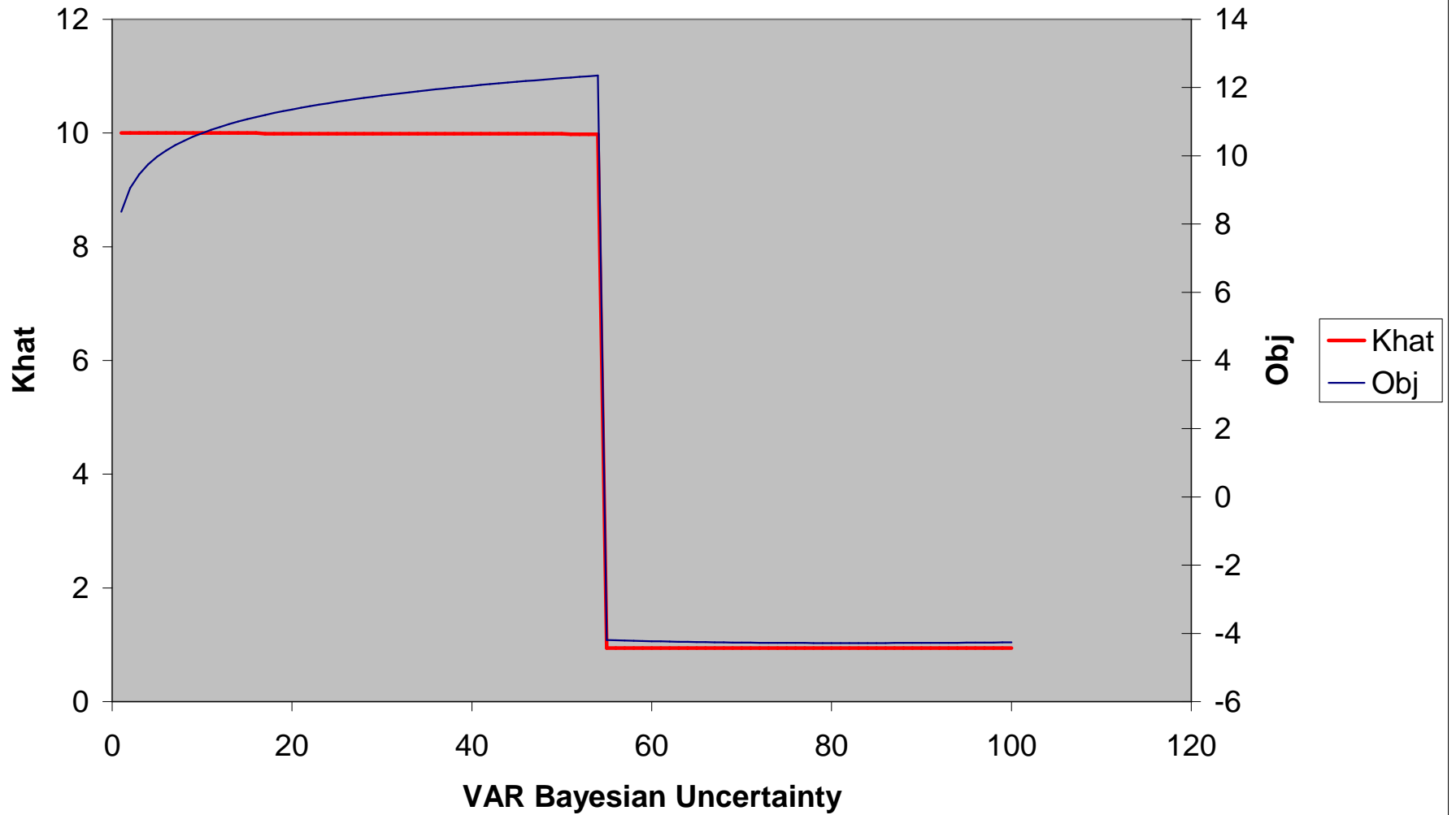
Data FOCE NONMEM VI
